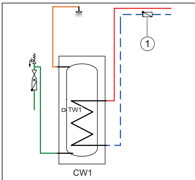
19. ábra Melegvíztároló
