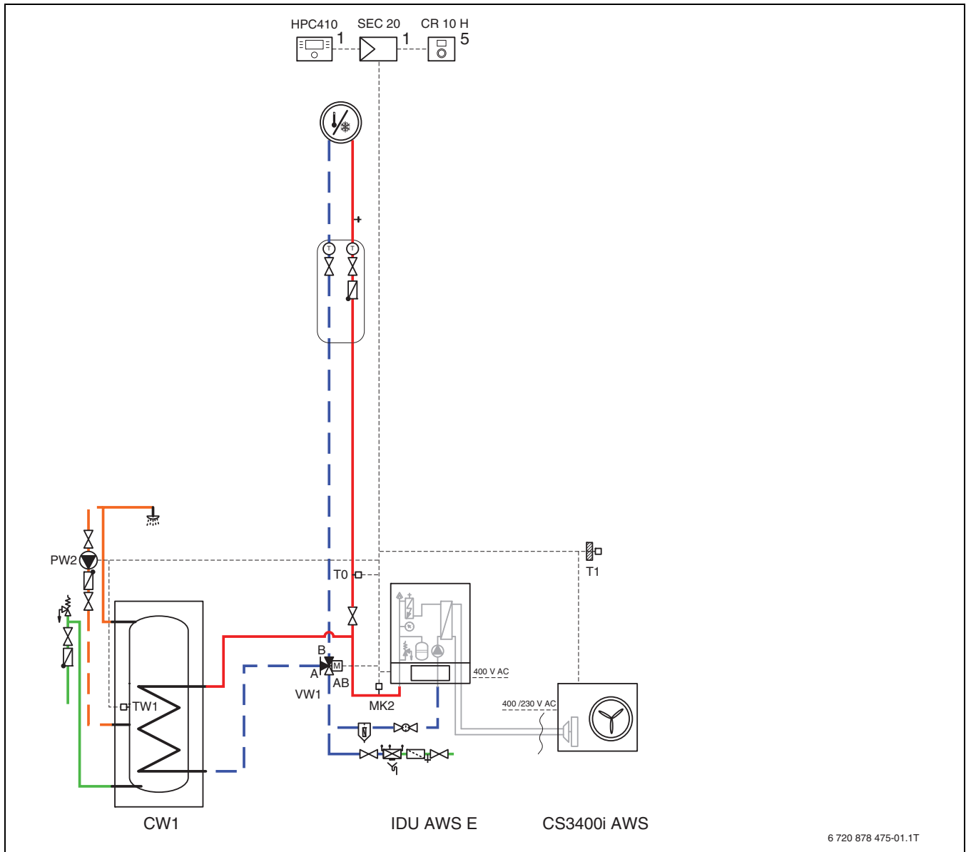
32. ábra Kültéri egység beltéri egységgel és egy fűtőkörrel
