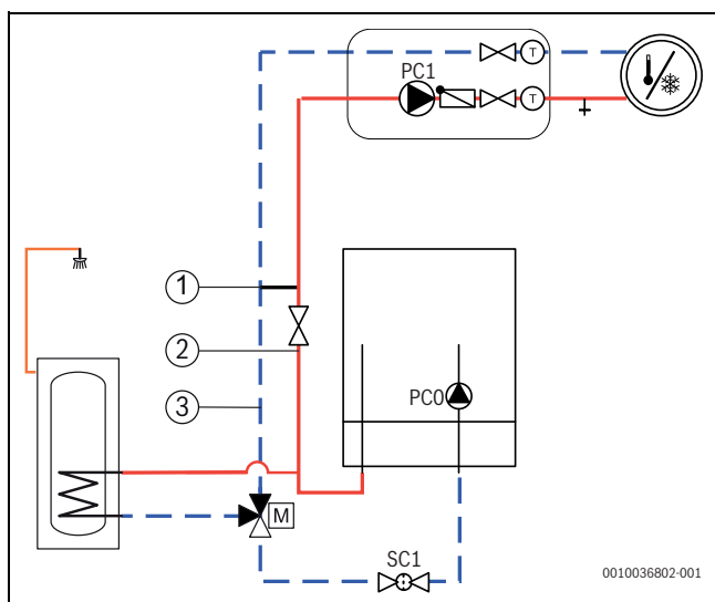
29. ábra Beltéri egység fűtőkörrel ésHVM körrel
