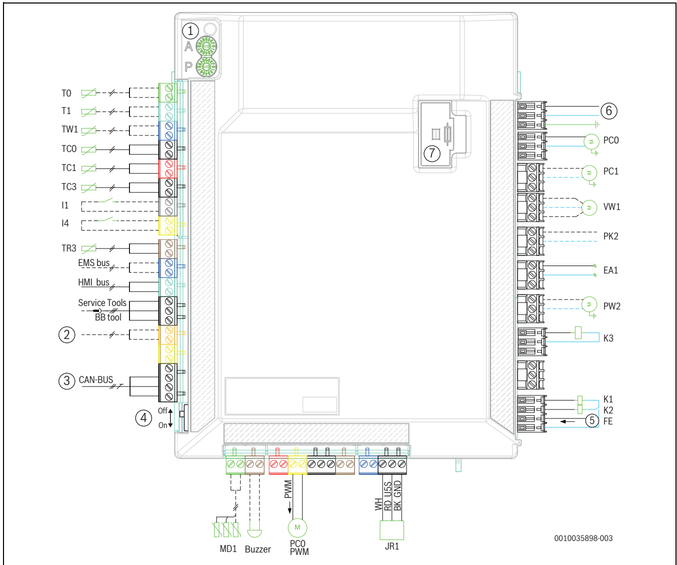
35. ábra A beltéri egység telepítói modulja
