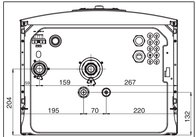
5. ábra Méretek és csatlakozások (csepegtetőtálca nélkül)
