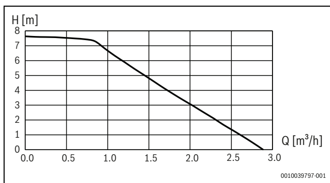
27. ábra Aprimer keringetőszivattyú (PCO) teljesítménygörbéje
